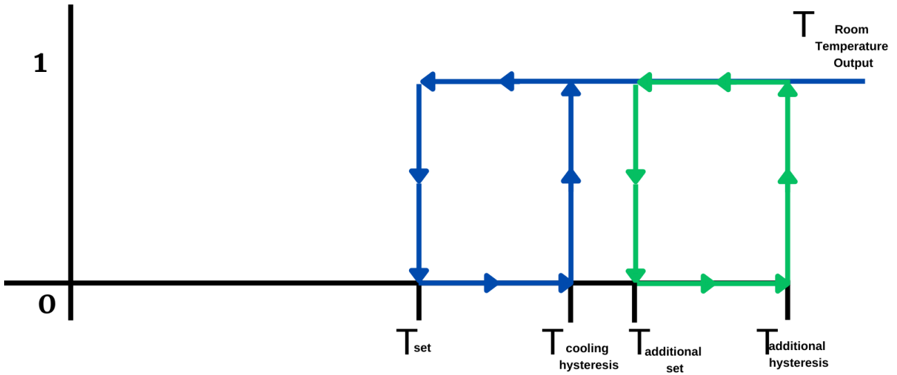
Soğutma için ek bölge histeresiz çalışması
