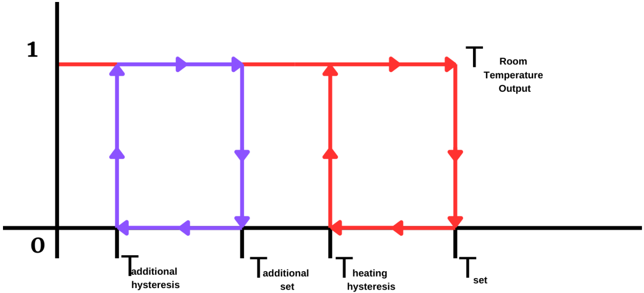
Isıtma için ek bölge histeresiz çalışması
